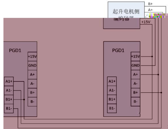
四线制编码器第二种接法
